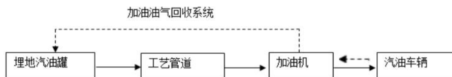
图 2.6-2 汽油加油工艺流程框图
