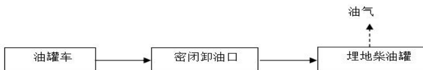
图 2.6-3 柴油罐车卸油工艺流程框图
