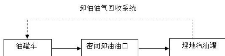
图 2.6-1 汽油罐车卸油工艺流程框图
