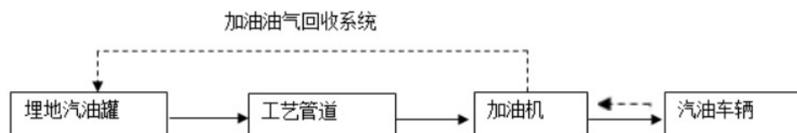
图 2.6-2 汽油加油工艺流程框图
