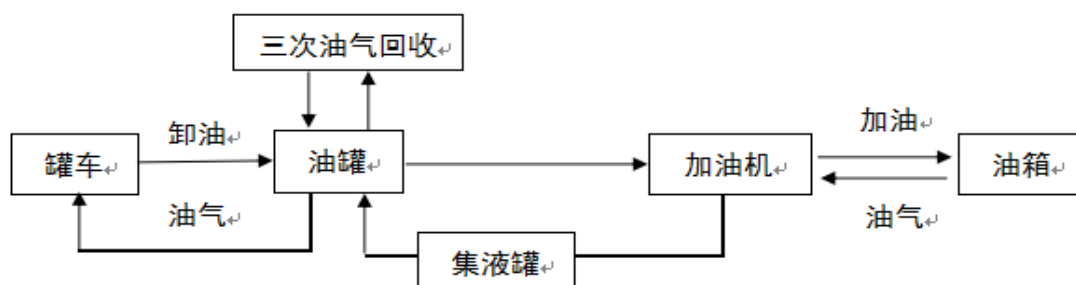
图 2.6-1 汽油卸油、加油、油气回收工艺流程图
