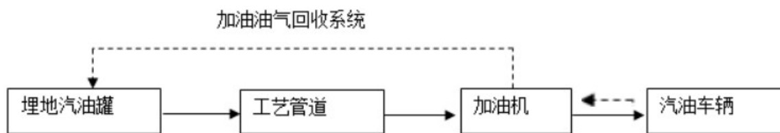
图 2.7-2 汽油加油工艺流程框图
