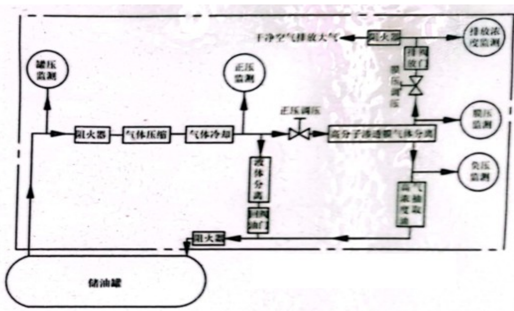
图 2.7-5 三次油气回收工艺流程图
