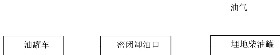
图 2.7-3 柴油罐车卸油工艺流程框图
